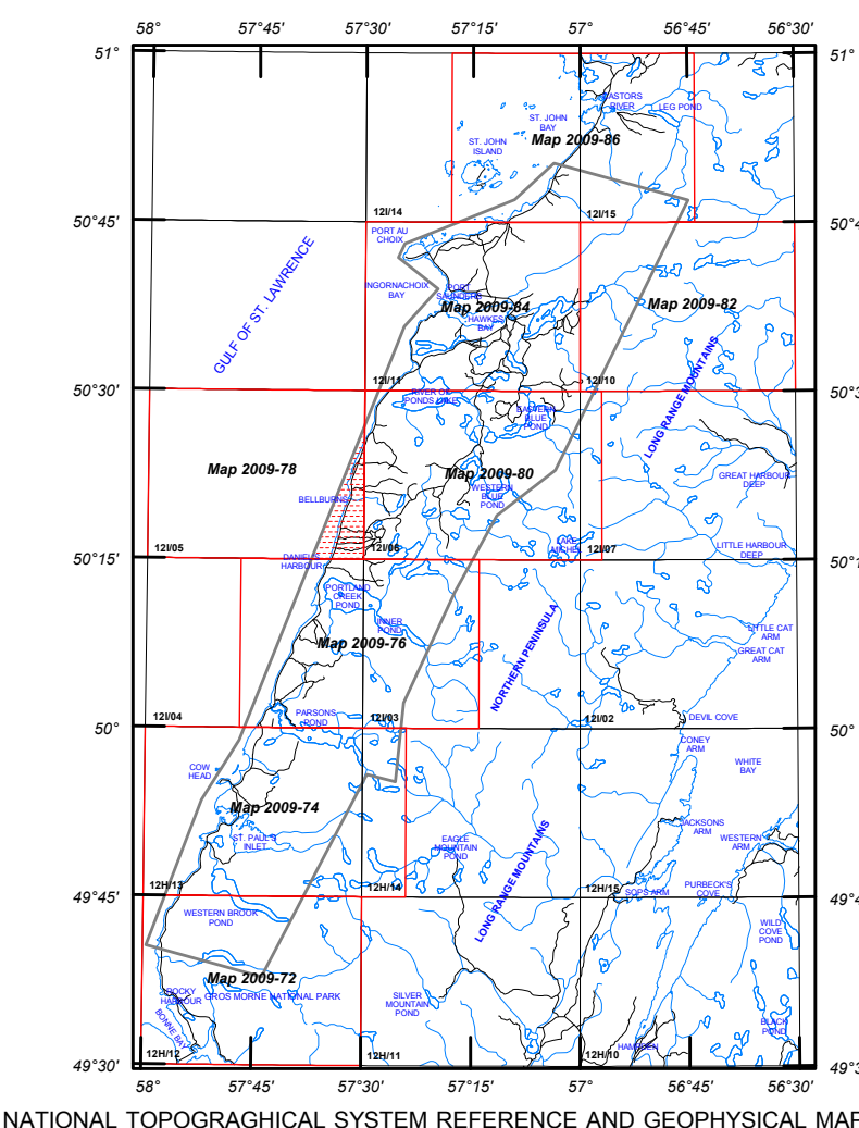
AEROMAGNETIC SURVEY - GROS MORNE TO PORT AU CHOIX AREA
