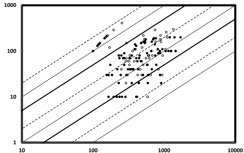
Zr (INAA) / ppm
