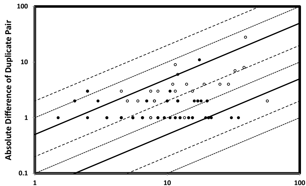
Cr (INAA) / ppm
