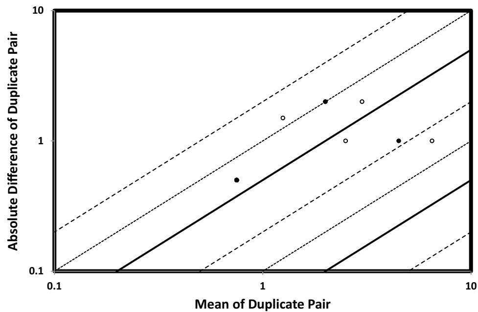
Mo (INAA) / ppm
