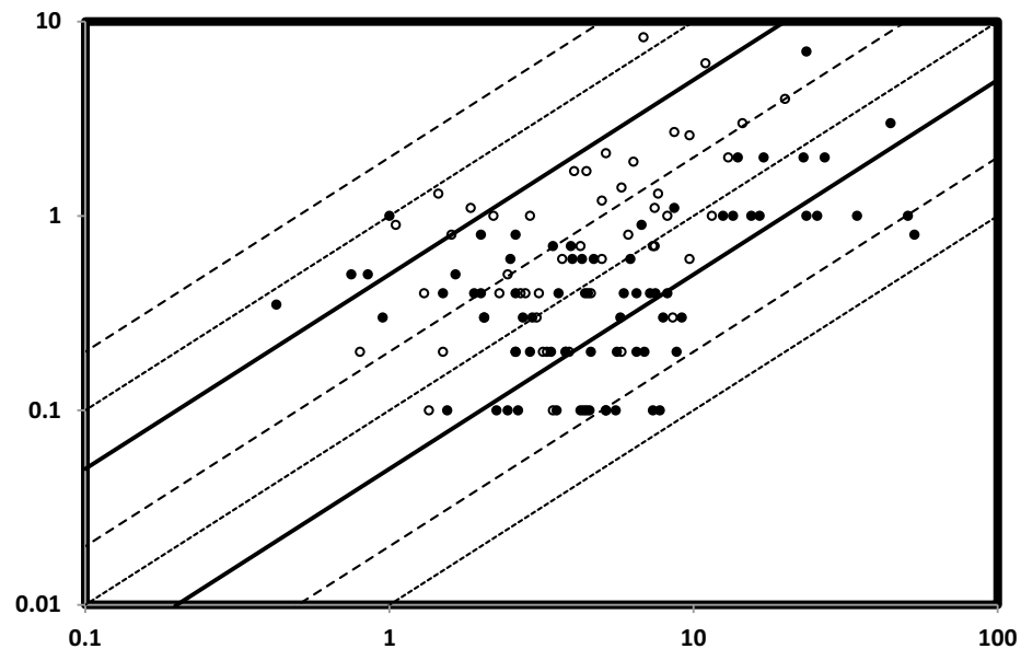
Au (INAA) / ppb
